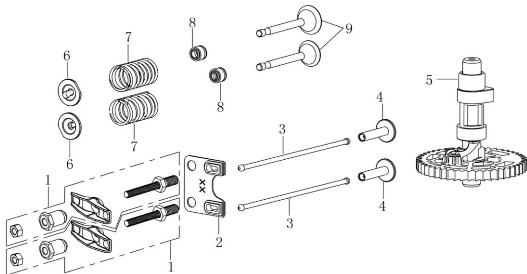
配气机构 (CAMSHAFT)
