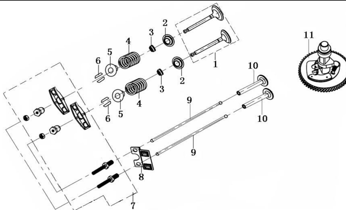
配气机构 (Valve)
