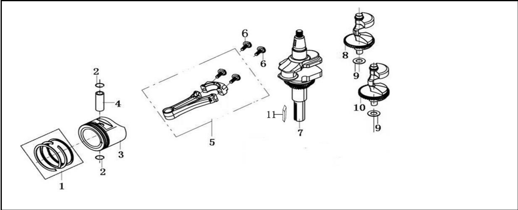
曲柄连杆（Crankshaft）
